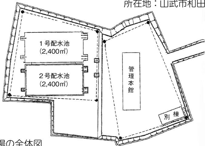
成東配水場の全体図
