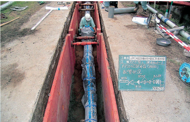
配水管改良工事
