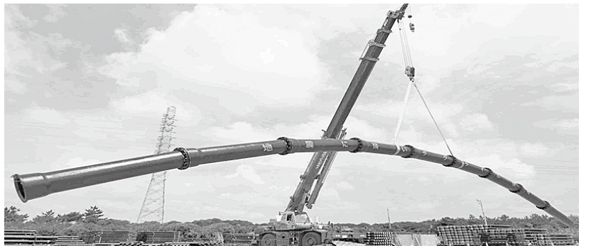
耐震性に優れた水道管（NS型ダクタイル鋳鉄管） 「一般社団法人日本ダクタイル鉄管協会」提供
